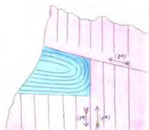
Fig. 1. Lorys theoretische Erklärung der Kalkkeile der Berneralpen.
